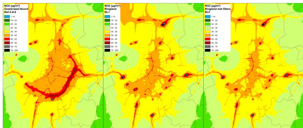
Figuur 6-50 NO 2 concentraties in 2020 voor het Oosterweel-Noord scenario (links), het Ringland scenario (midden) en het Ringlandscenario met bijkomende filtering (rechts). Bron: VITO, 2015.
