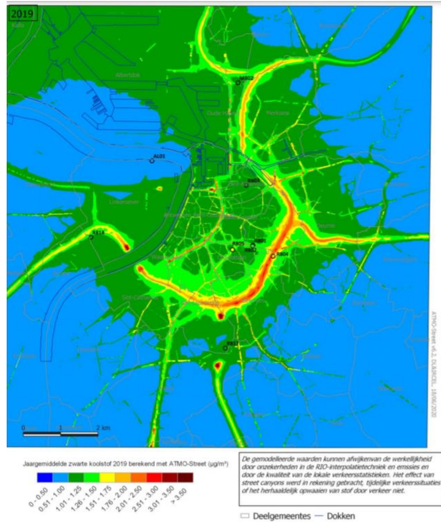
Figuur 6-39 Jaargemiddelde EC-concentratie in 2019 (bron: VMM)
