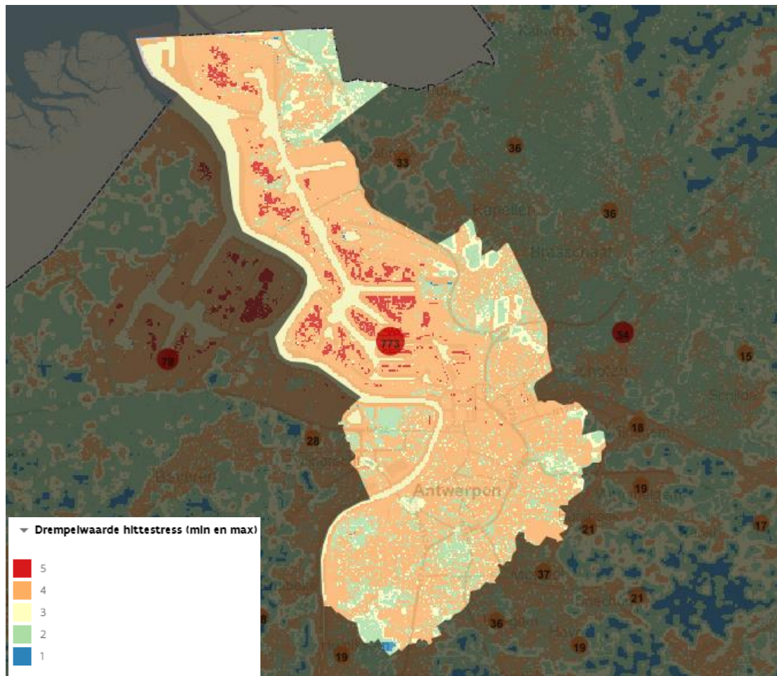
Figuur 6-41 Drempelwaarde Hittestress klimaatscenario 2030 (Bron: VMM). Legende bij de drempelwaardes die overschreden worden voor dagmaximum en dagminimum gevoelstemperatuur tijdens een extreme hittedag met een terugkeerperiode van 20 jaar. Dit wordt weergegeven in 5 klassen, waarbij vanaf score 4 (oranje) ernstige gezondheidsschade te verwachten is.
