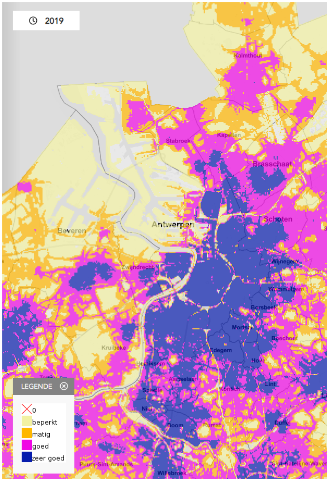
Figuur 6-15: voorzieningenwaarde
