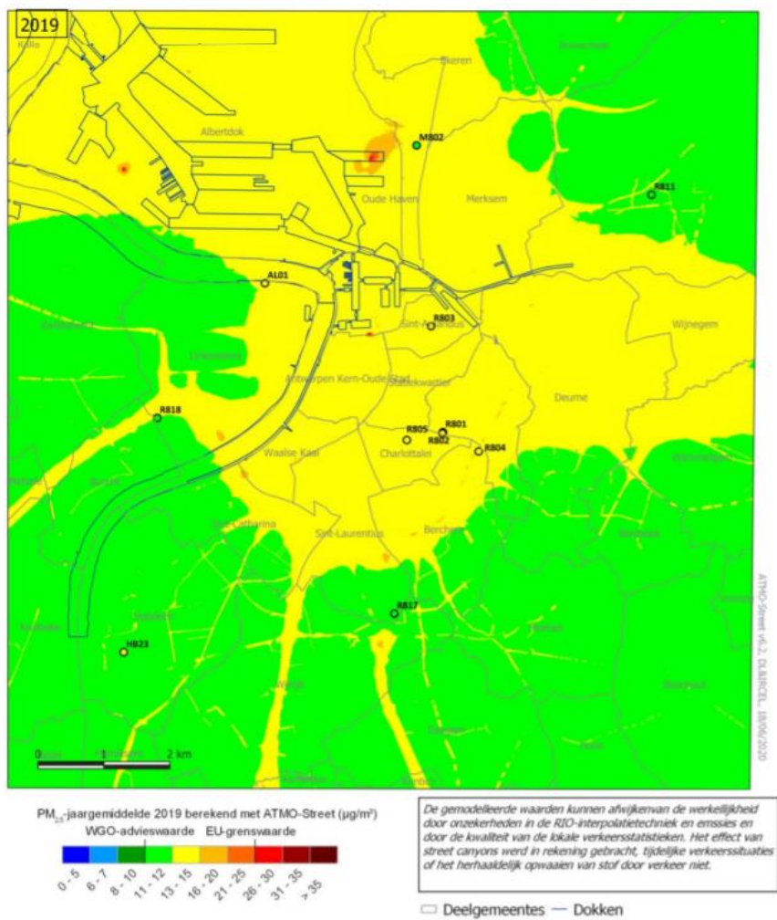
Figuur 6-38 Jaargemiddelde PM 2.5 -concentratie in 2019 (bron: VMM)
