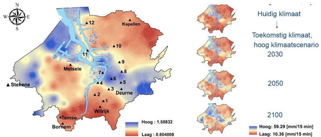
Figuur 6-32 Ruimtelijke variatie in de piekneerslag in Antwerpen en omgeving, en de berekende toekomstige evolutie ervan in een wijzigend klimaat (Neerslagstudie Antwerpen, KU Leuven, 2014)
