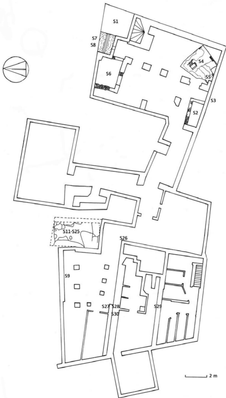
Figuur 8. Sporenplan
