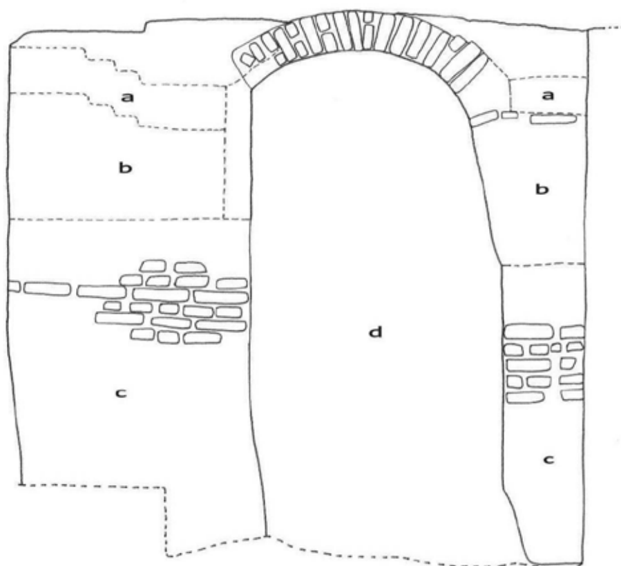
Figuur 18. Lengteprofiel van afvalput S4 a: gewelf afvalput b: oostelijke wand afvalput c: oostelijke wand storthelling d: stortvlak
