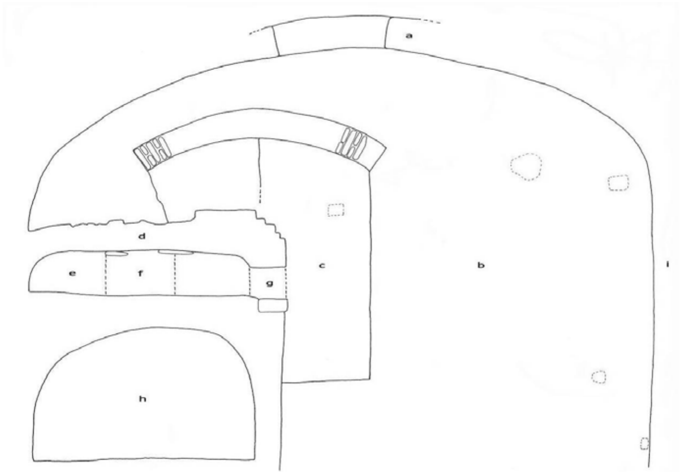
Figuur 26. West-oost doorsnede van oven S7 en keldervertrek S1
