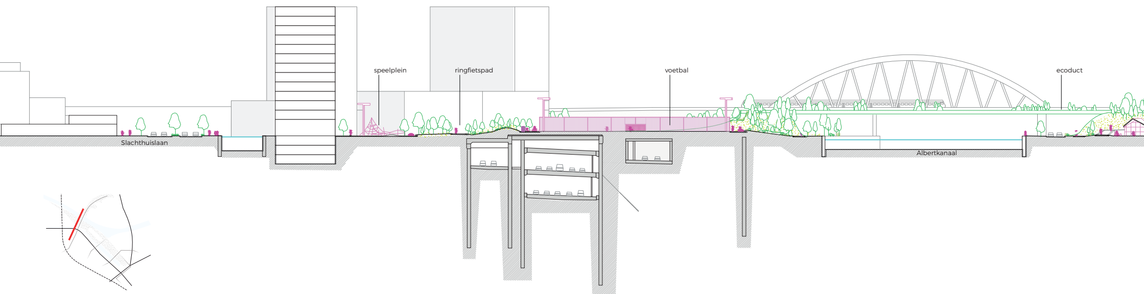
doorsnede kap Dam
