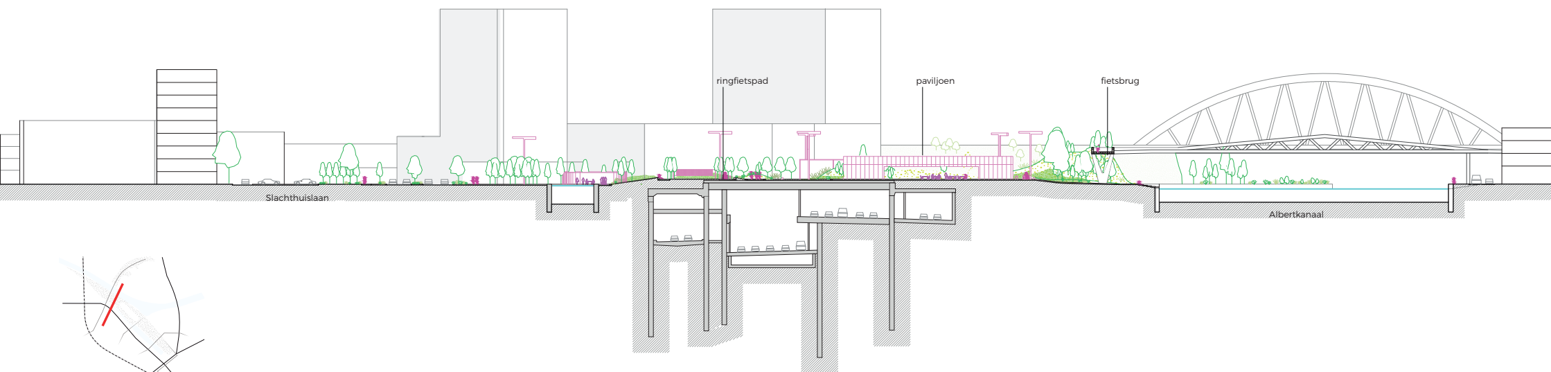
doorsnede kap Dam
