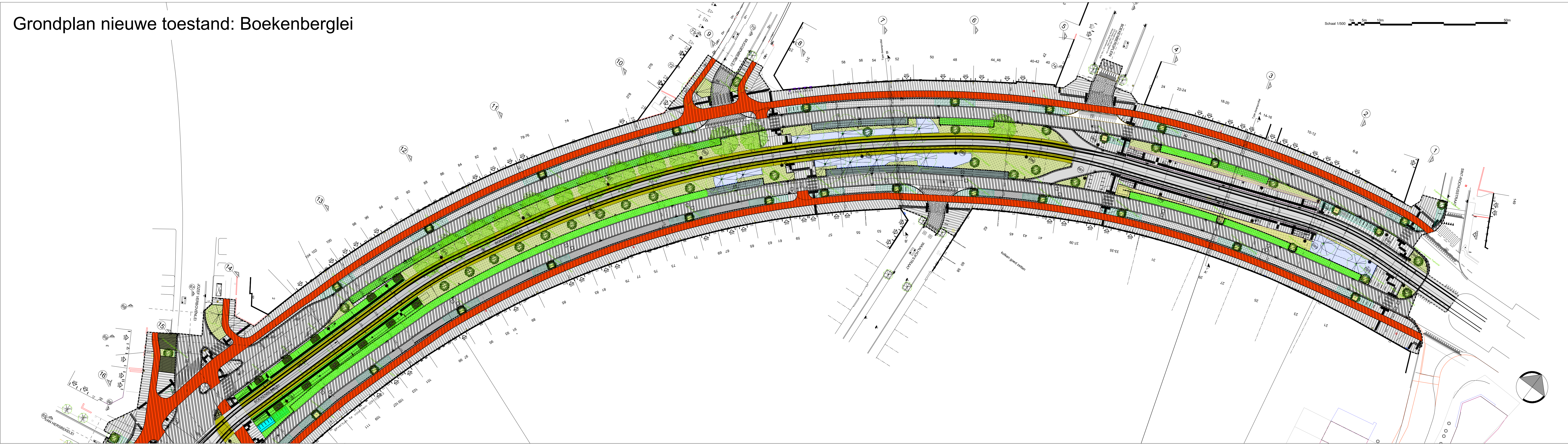
Grondplan nieuwe toestand: Boekenberglei
