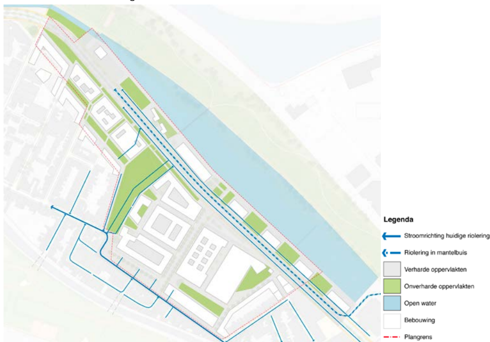
Bestaande droogweerafvoer (Startadvies Slachthuisite, Riolink NV).
