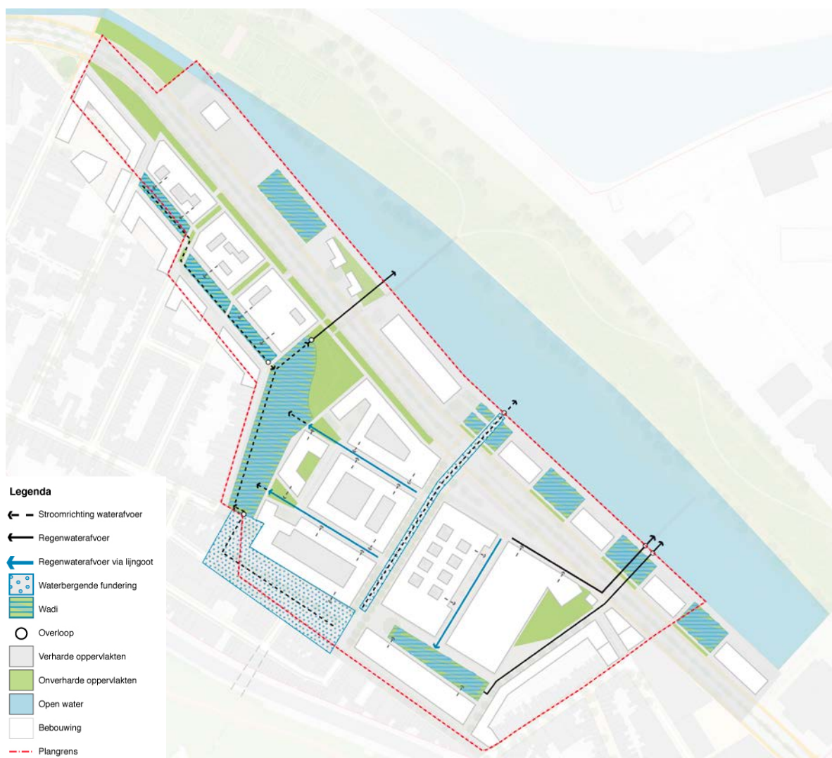
Voorstel hemelwaterafvoer
