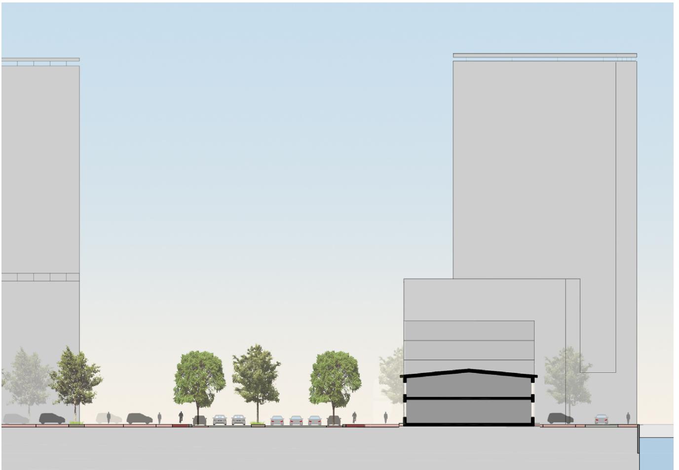
snede over Slachthuislaan/Lobroekkade-zuid met verkelinde footprint voor de kade-bebouwing
