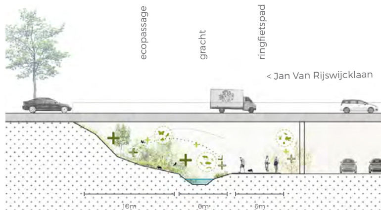
Principe van brede onderdoorgangen bij de radiaalbruggen (groene verbinding, gracht, fietspad)
